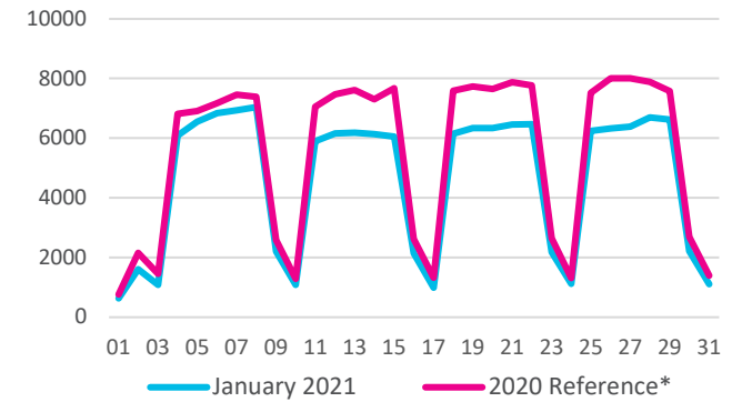
M1 J2 - J3 HGV 24H Flow
