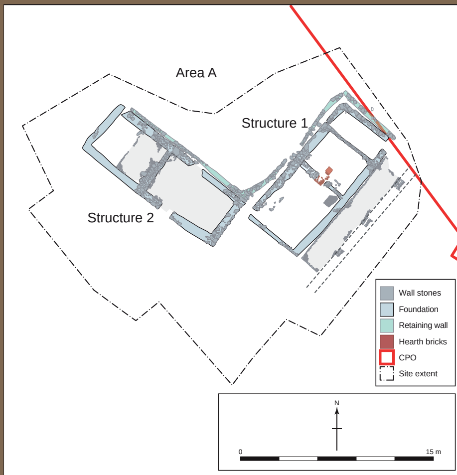
Plean de na struchtúir 1 agus 2 ag Eanach1, Contae na Gaillimhe. (Na hiomhaí uilig: Headland Archaeology (Ireland) Teo)
