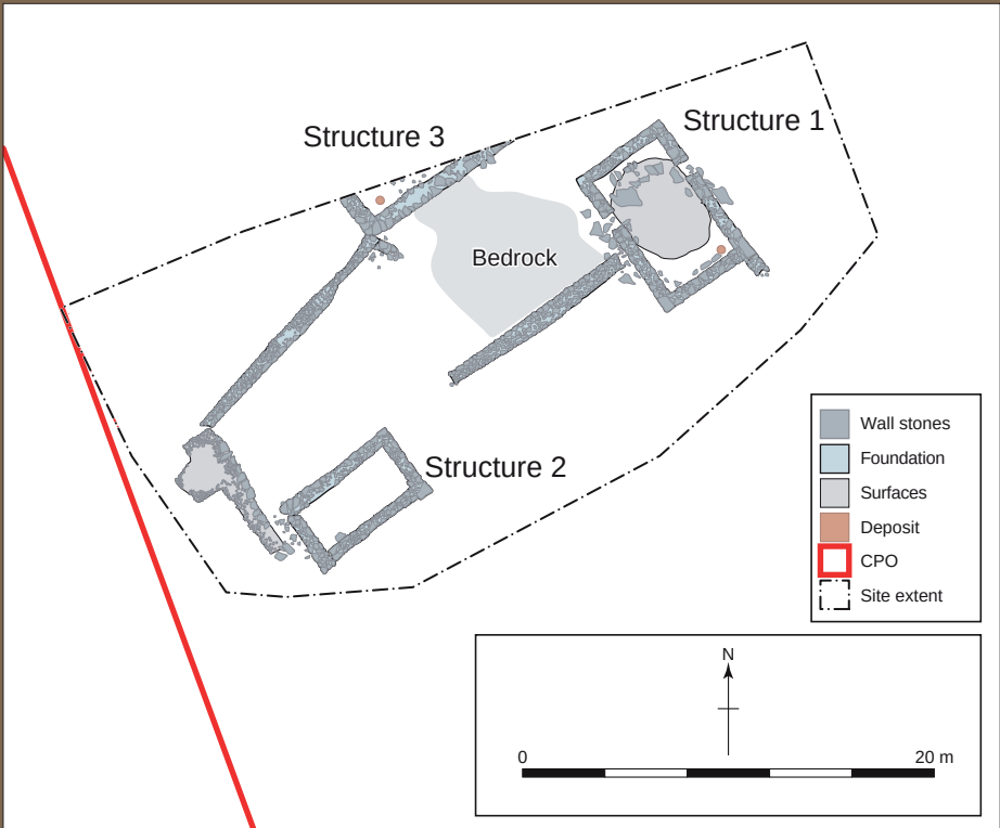
Plean de struchtúir 1-3 ag Cill Scéithe 4, Contae na Gaillimhe.
