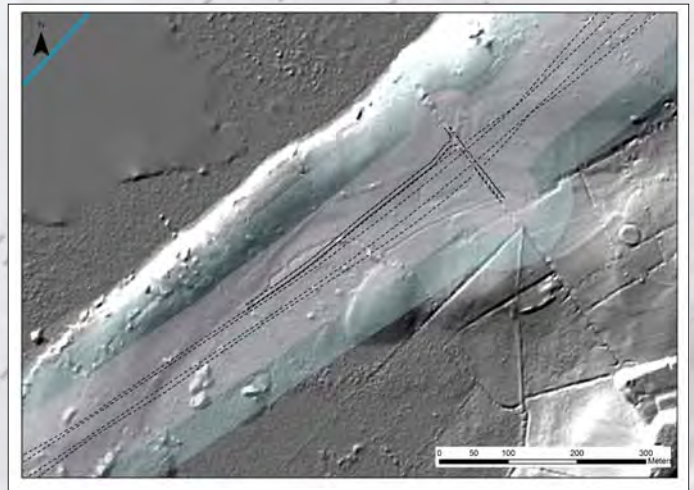
Bealach molta do scéim bhóthair N4 Cora Droma Rúisc – Dromad (líne bhriste), maoláin 50m agus 100m (scáthaithe), agus íomhá LiDAR.
