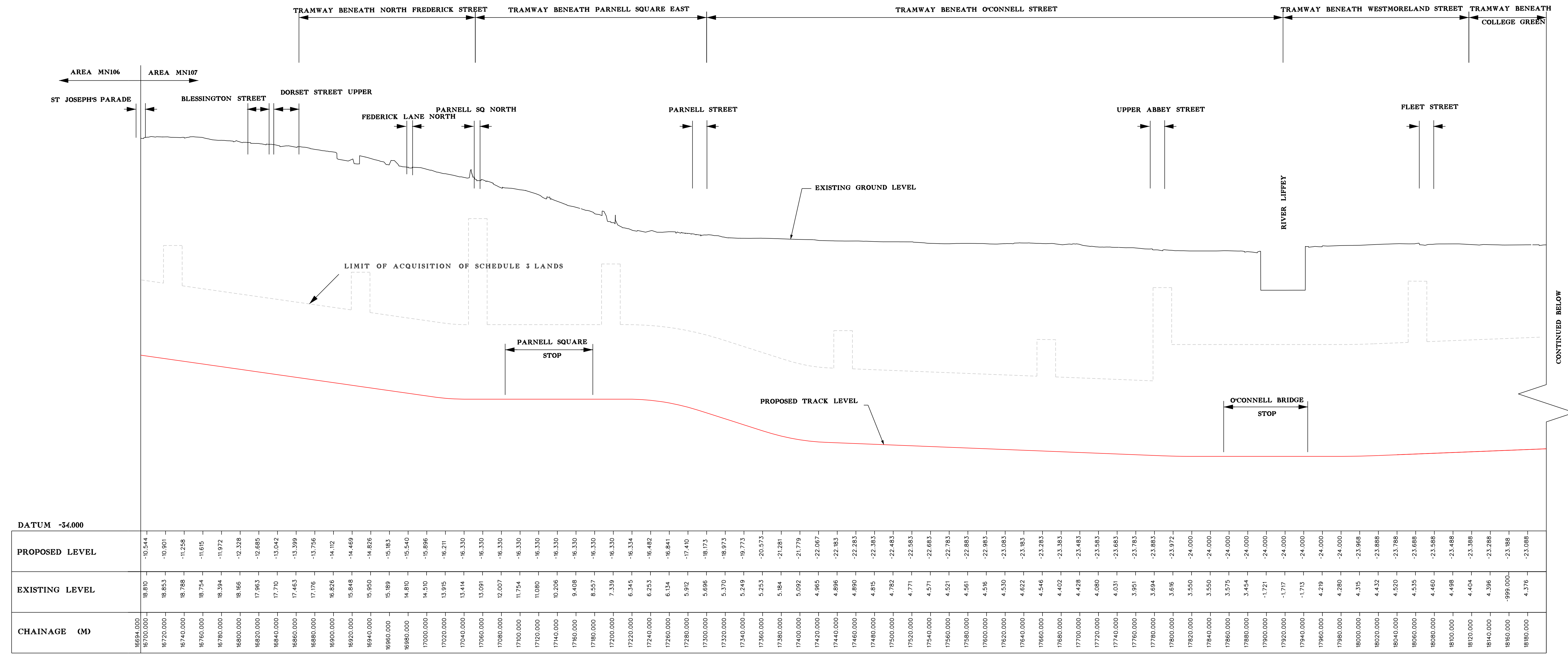
LONGITUDINAL SECTION SCALE: HORIZ 1:2000 VERT 1:250
