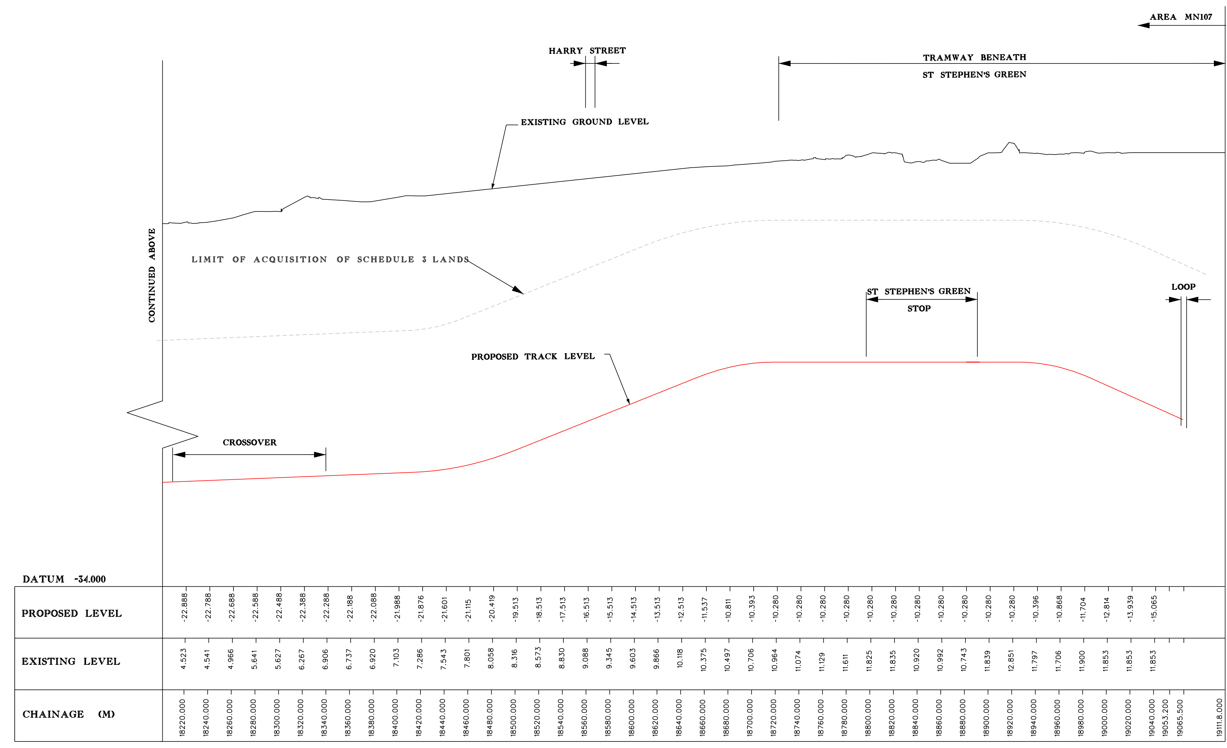
LONGITUDINAL SECTION SCALE: HORIZ 1:2000 VERT 1:250
